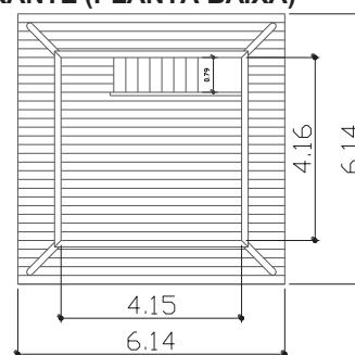
FIGURA 144 – MIRANTE (PLANTA BAIXA)
