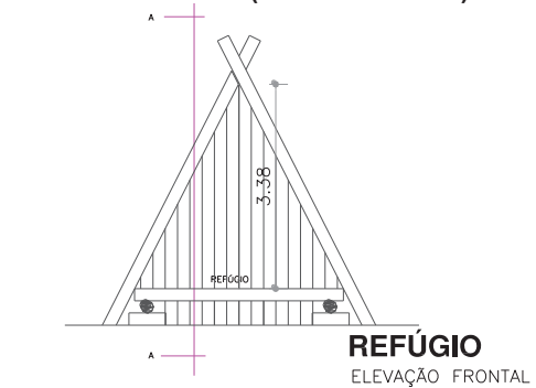
FIGURA 152 – REFÚGIO (VISTA E CORTE)
