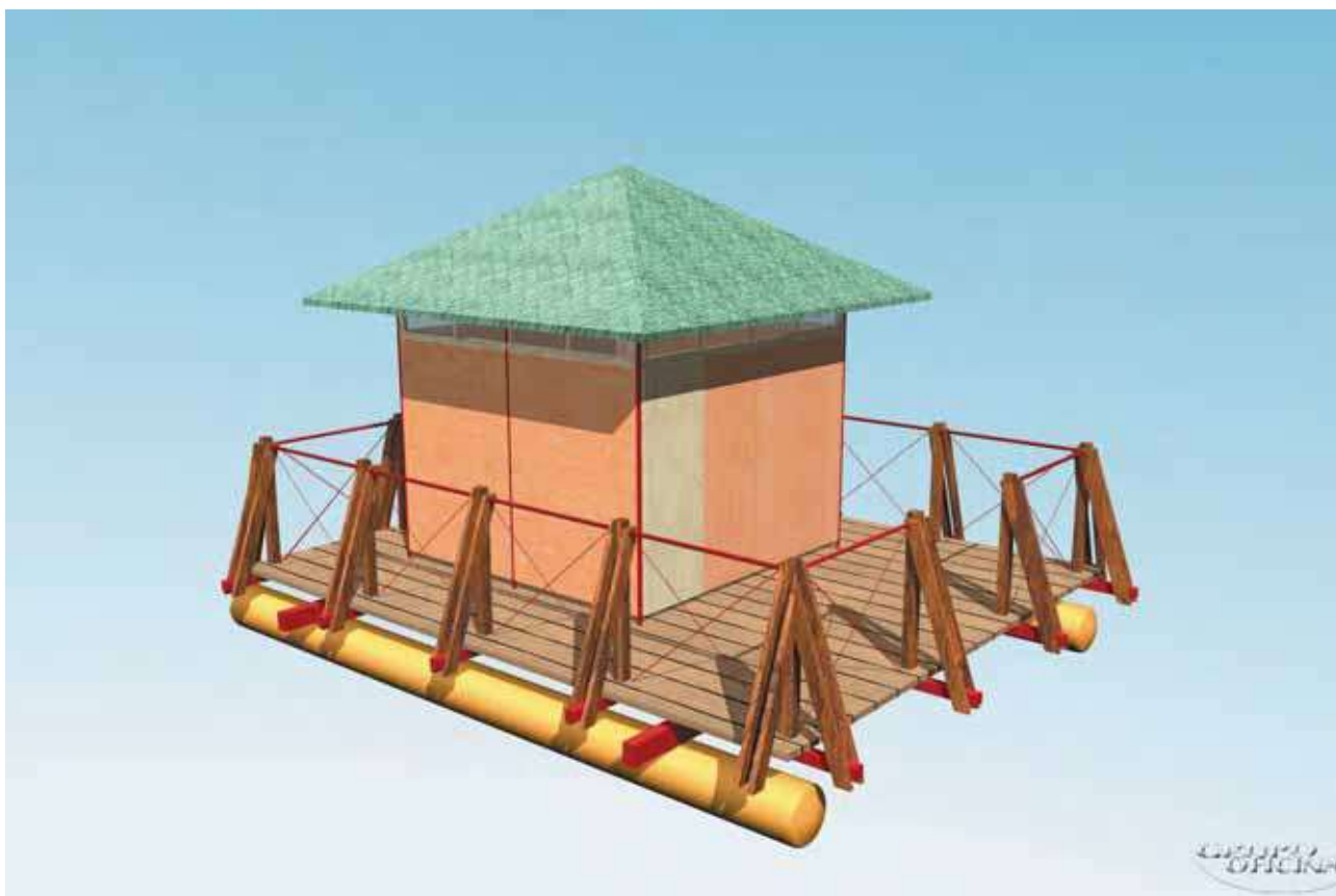
FIGURA 113 - PLATAFORMA FLUTUANTE: MÓDULO DE APOIO A EMERGÊNCIAS
