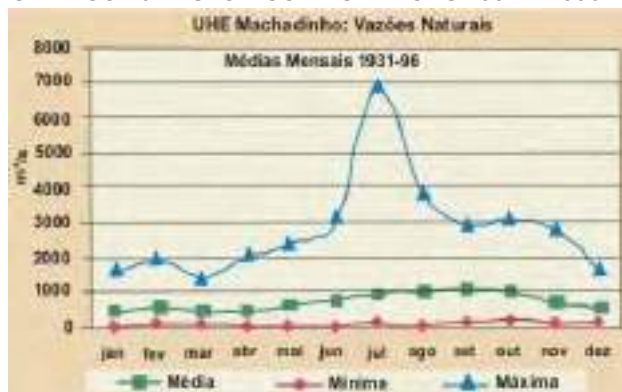
GRÁFICO 10: HISTÓRICO DAS VAZÕES 1931 A 1996
